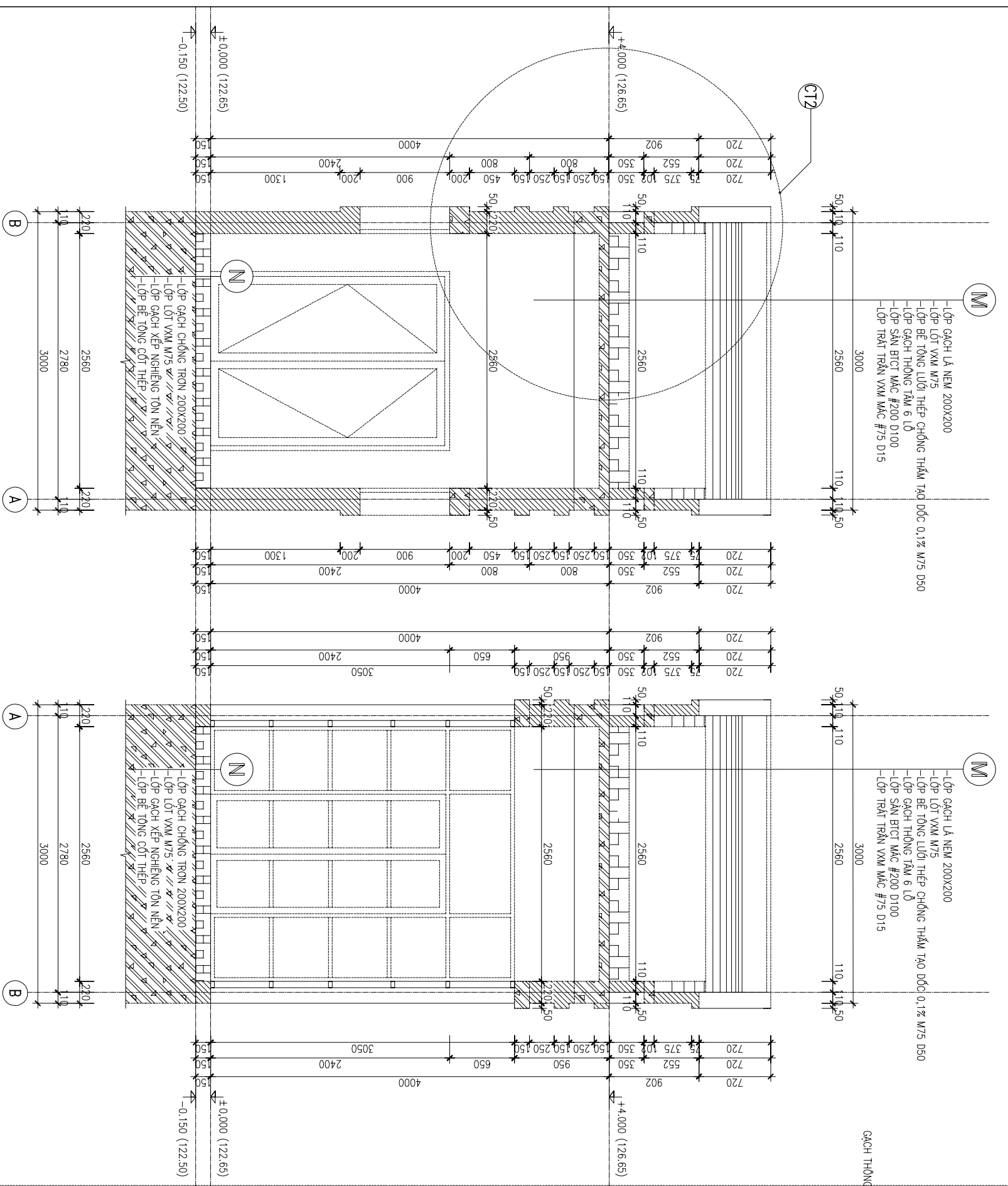
MẶT CẮT 2-2
